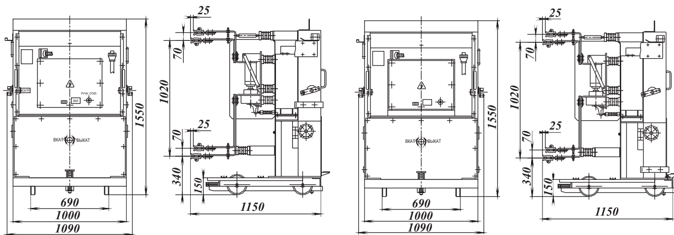
Выкатной элемент для КРУ серии К-XV
