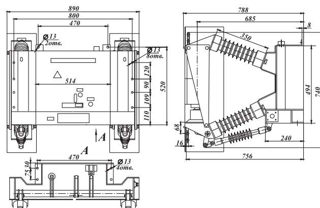
ВБД-27,5-25/1600 УЗ
