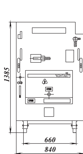
Выкатной элемент для КРУ серии K-XII, K-XXVI
