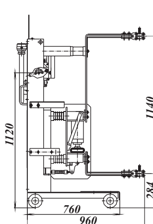
Выкатной элемент для КРУ серии ST-7
