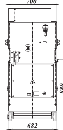
Выкатной элемент для КРУ серии ST-7
