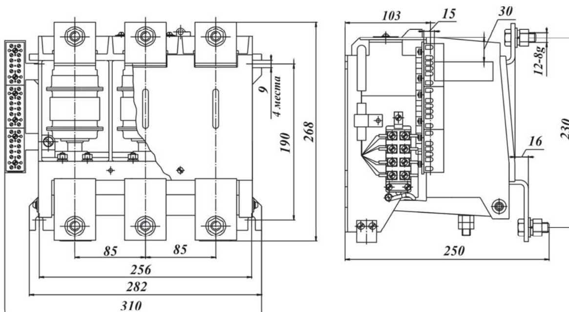
1. Контактры типа КВТ2-1,14 с выводами “вверх-вниз”, с клеммной колодкой.
