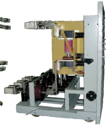
ВБЭ-10-31,5(40) для яч. К-33М, К-37
