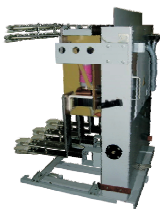
ВБЭ-10-31,5(40) для яч. К-ХХVII, К-ХV
