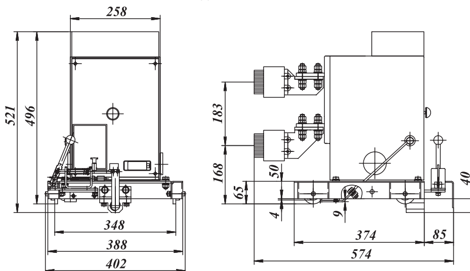
4.6 Габаритно-присоединительные размеры выкатного элемента ячейки КРУ типа EJF(чешка) с вакуумным выключателем ВВА-1,14
