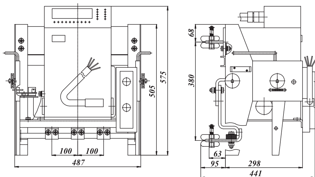
4.3 Габаритно-присоединительные размеры выкатного элемента ячейки КРУ типа АРУ-30 (Польша) с вакуумным выключателем ВВА-1,14
