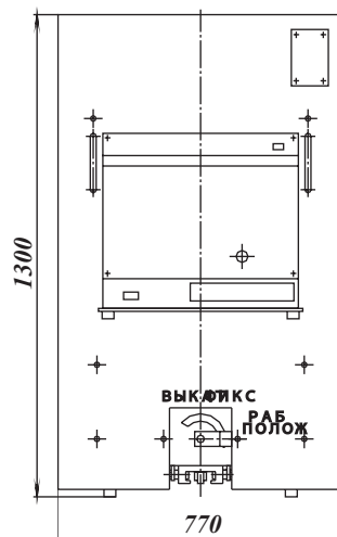
Выкатной элемент для КРУ серии ST-7
