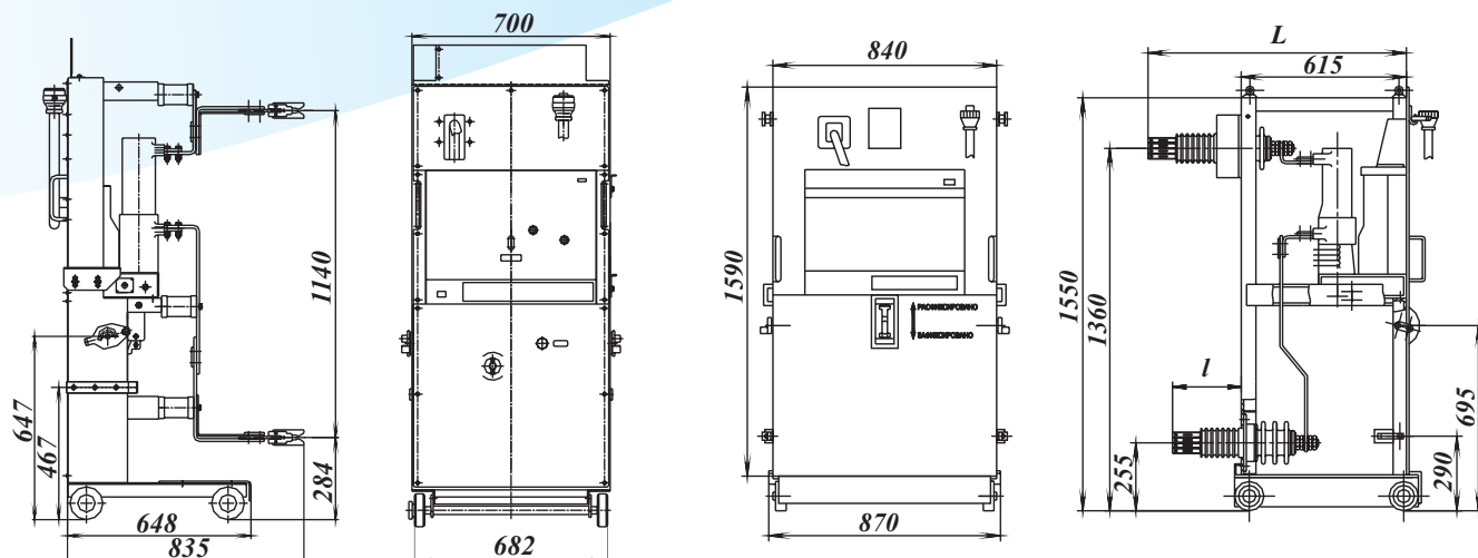
Выкатной элемент для КРУ2-10 нижн вал с ВБ (для замены ВМПЭ-10 и ВМПП-10)
