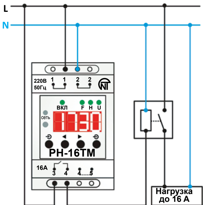
Схема подключения
