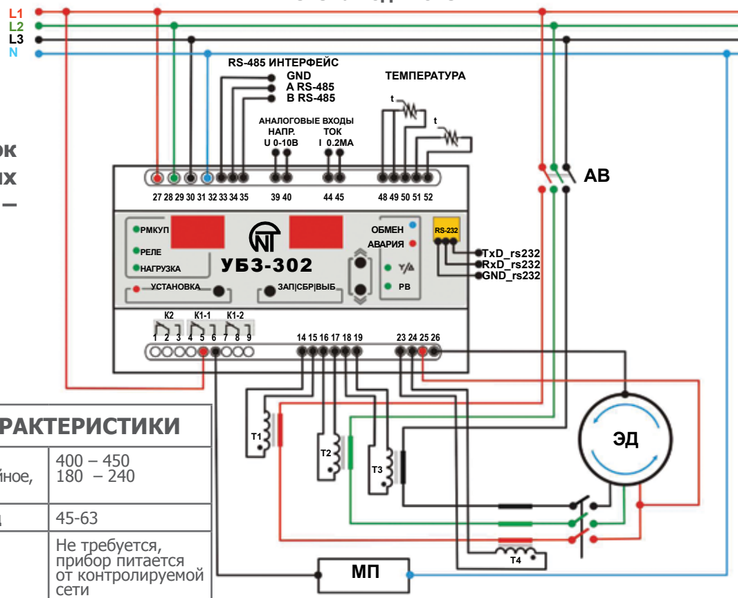
Схема подключения
